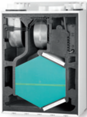
Logavent HRV 21: optimierte Wärmeisolierung durch Innenkonstruktion aus EPP-Schaum
